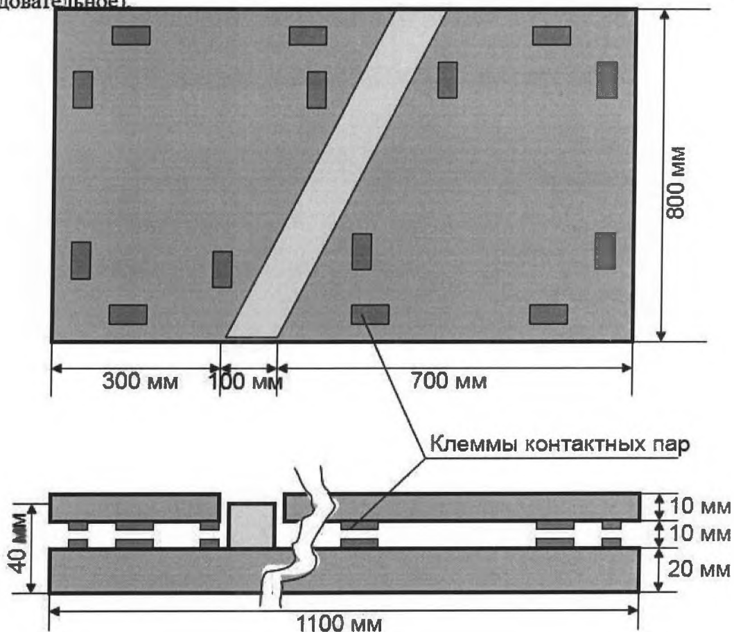
Рисунок № 1. Схема контактной финишной площадки.
