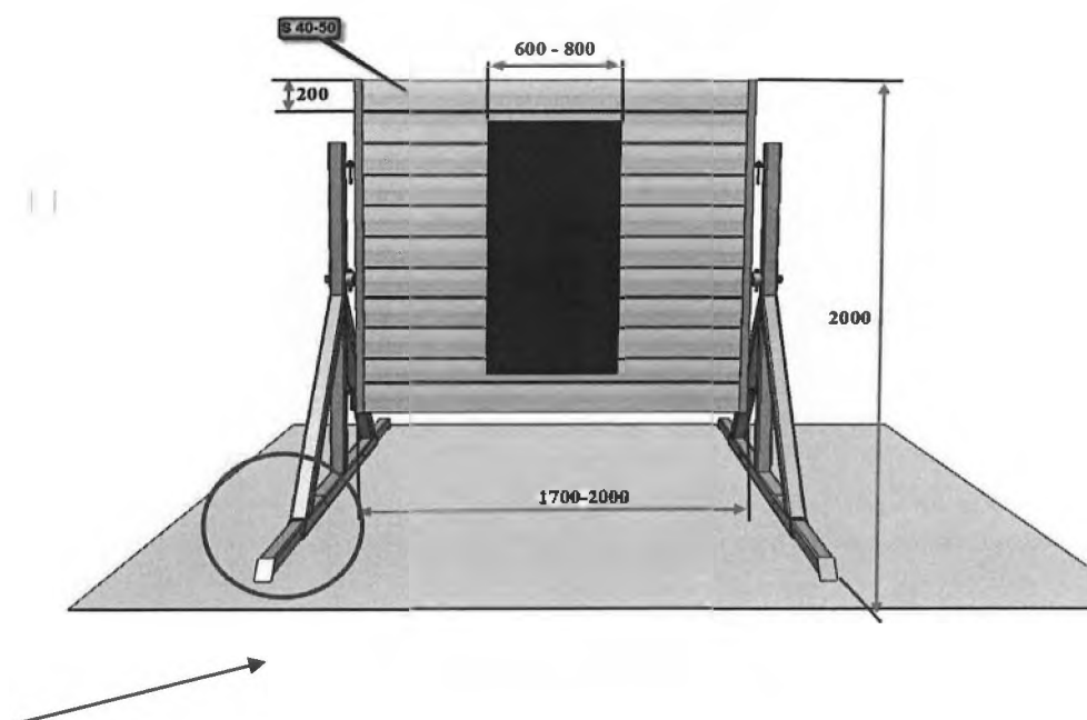
Рисунок № 1. Схема спортивного снаряда «забор».
