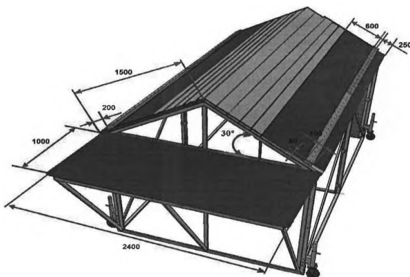
Рисунок № 1. Схема спортивного снаряда «Домик».
