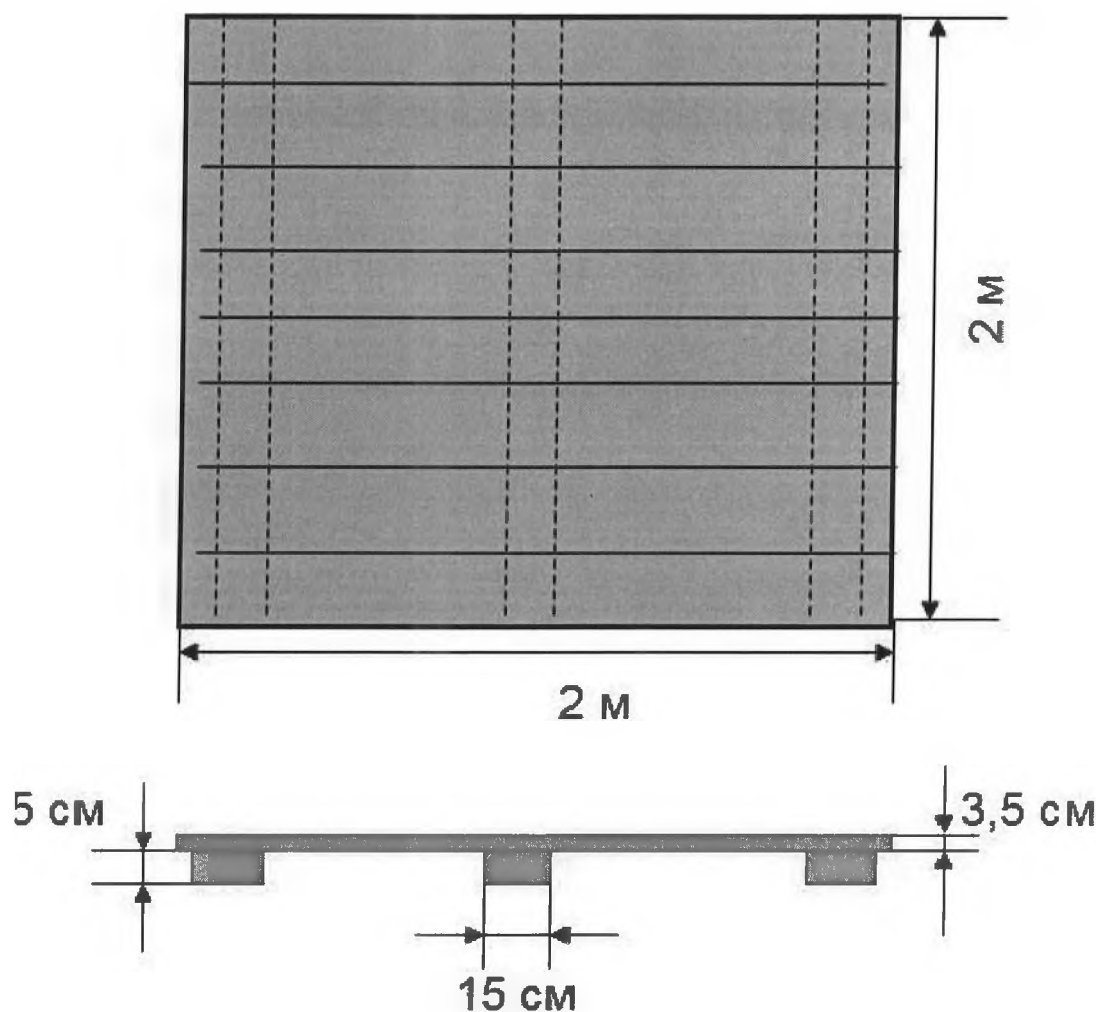
Рисунок № 1. Схема спортивного оборудования «щит».
