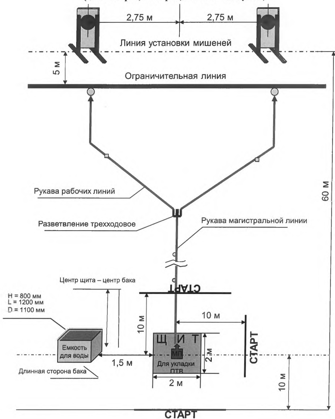
Рисунок № 1. Схема размещения оборудования в спортивной дисциплине «боевое развертывание».
