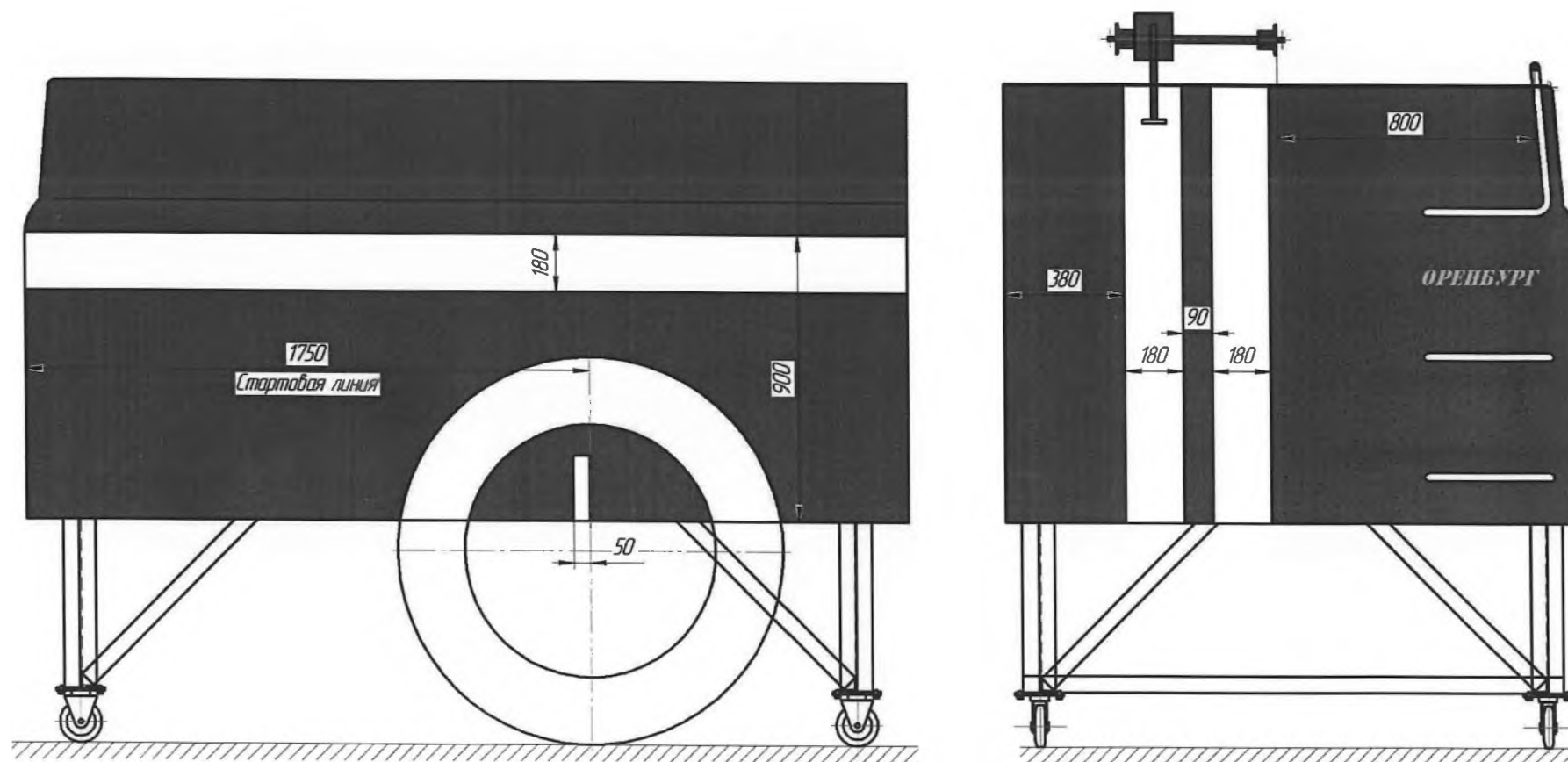
Рисунок № 1. Общий вид макета АЦ.
