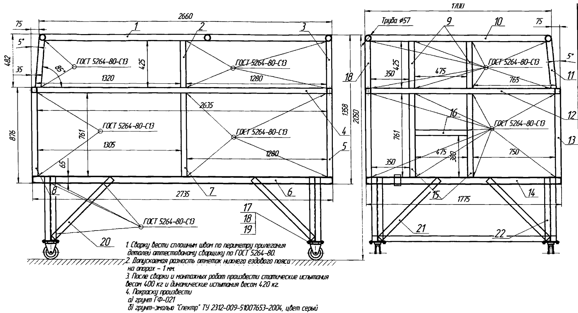
Рисунок № 4. Вид макета АЦ сбоку.
